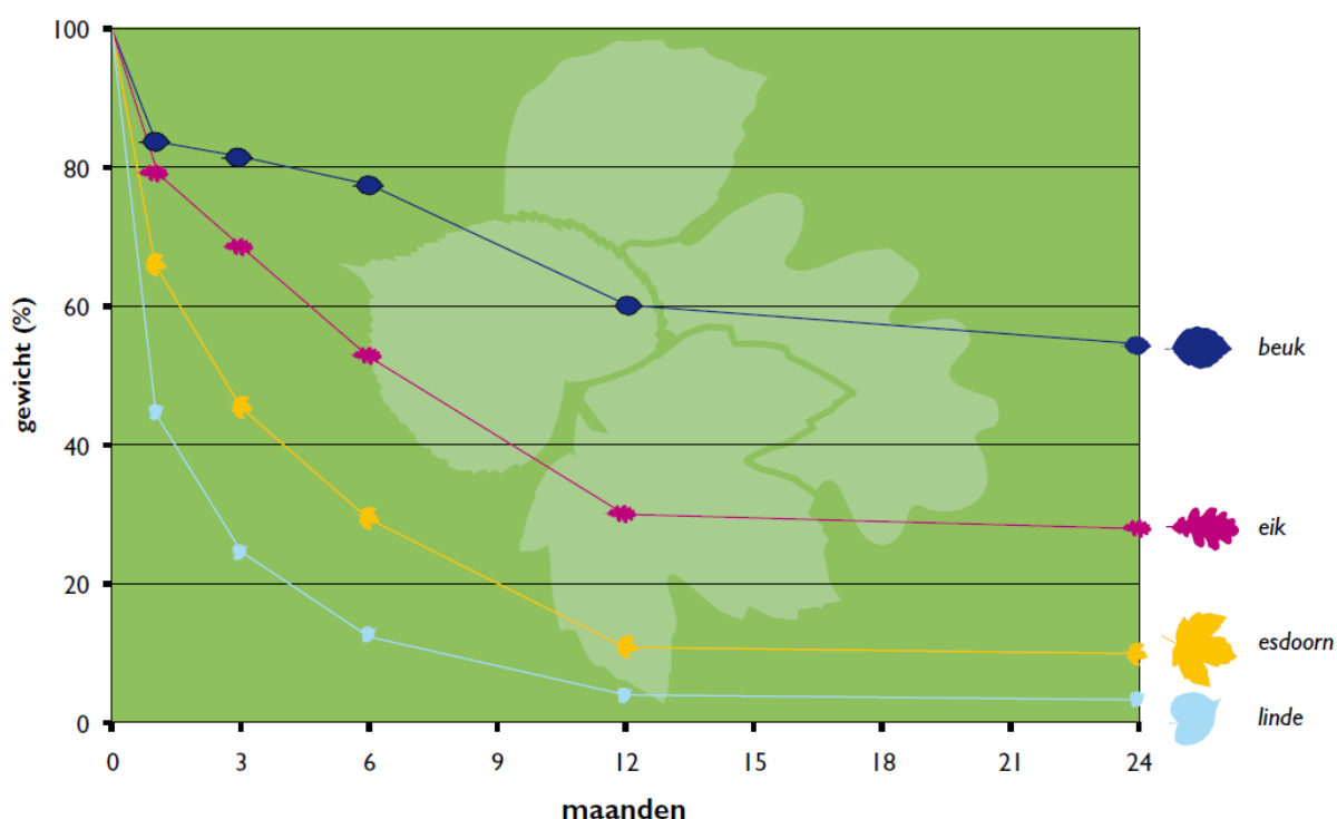
Figuur 3.5 Soortgebonden verschillen in afbraaksnelheid van bladstrooisel in een experiment waarbij strooisel van verschillende loofboomsoorten werd ingebracht in een dennenbos op arme zandgrond (Muys 1993).
